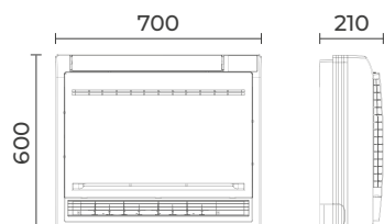
KL035-A1 / KL050-A1
